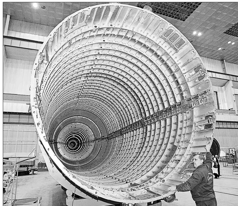
Внутрішній вигляд майбутнього ракетноносія, створеного на Південному машинобудівному заводі ім. А. М. Макарова
