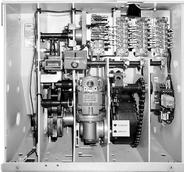
Такий вигляд має високовольтний вакуумний вимикач
