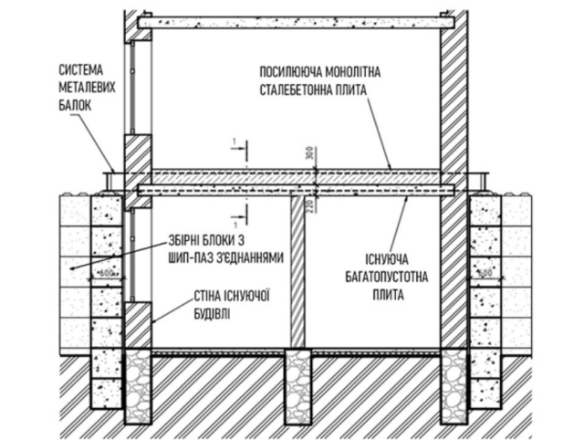
Підсилення перекриття та несучих конструкцій, що спираються на колони та бетонні або залізобетонні блоки
