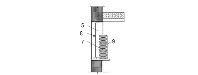
Заповнення віконного прорізу мішками з ґрунтом (піском)
