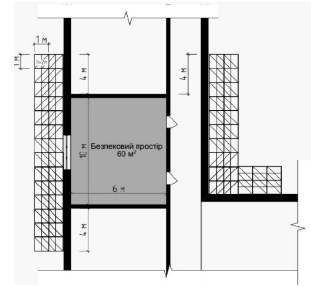
Захист віконних прорізів Заповнення віконного прорізу ґрунтом
