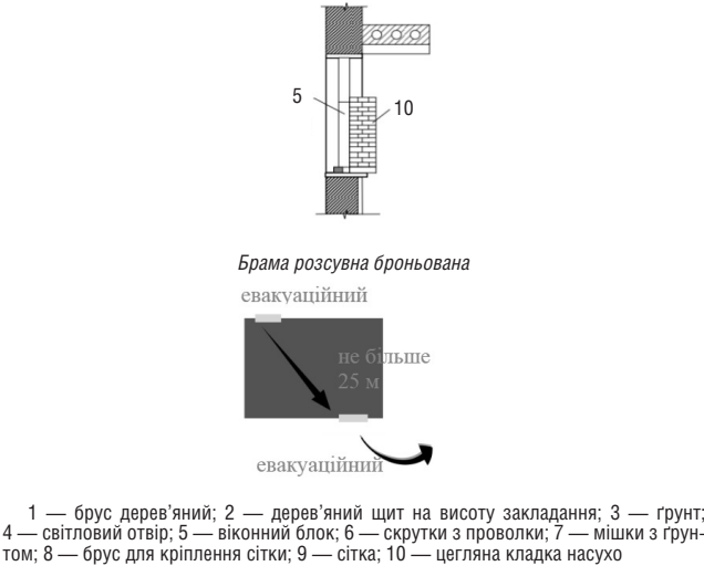
Заповнення віконного прорізу цегляною кладкою насухо
