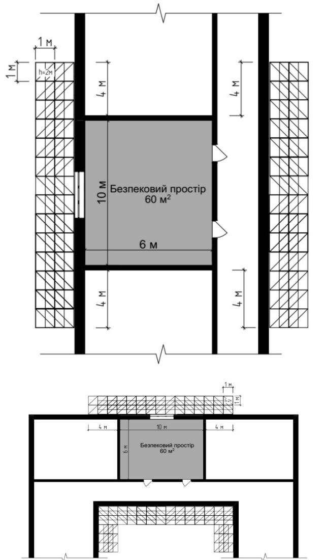
Додаток до Порядку ЗРАЗКИ основних інженерно-технічних рішень щодо створення захищених просторів Встановлення габіонів, наповнених сипучими матеріалами
