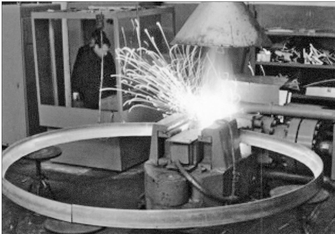
Ось так відбувається контактне стикове зварювання плавленням
