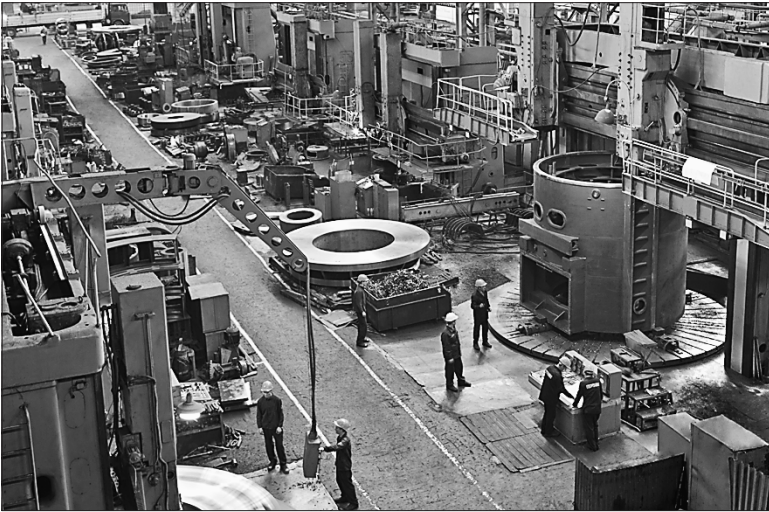
Крупномеханічний цех заводу «Електроважмаш»
