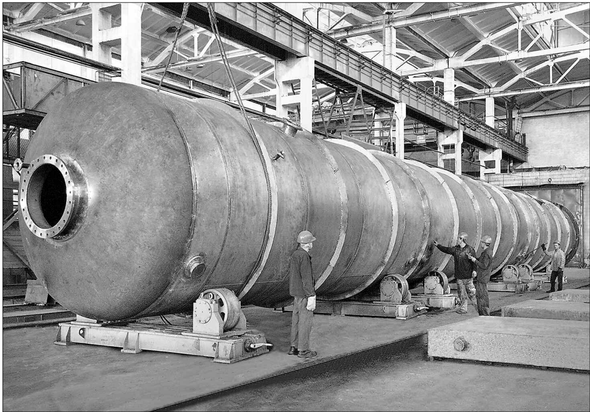
Сумські машинобудівники готують до відправлення дистиляційну колону, виготовлену на замовлення турецької компанії «Soda Sanayi»
