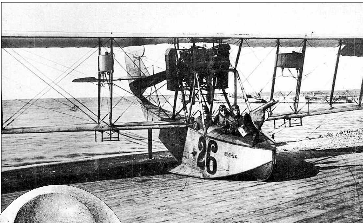
Літаючий човен М-9 Дмитра Григоровича на Балтійському флоті
