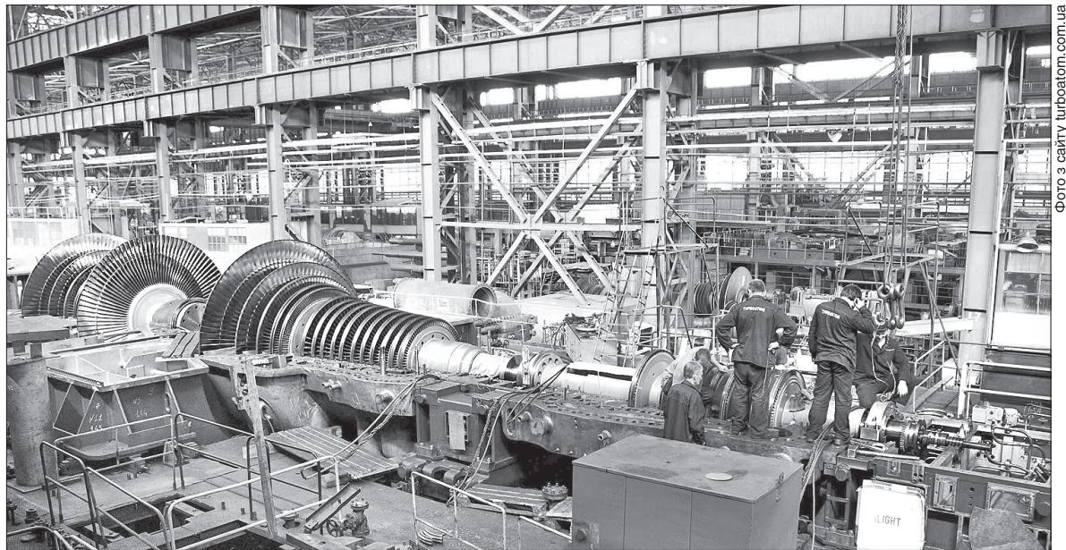
Збирання роторів на харківському ПАТ «Турбоатом», яке є дуже важливим підприємством в Україні
