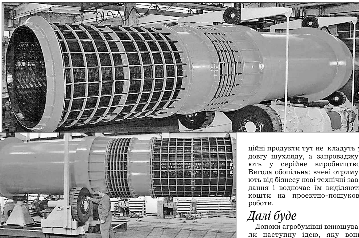
Ці потужні сучасні «динозаври» називаються скруббер-бутари і використовуються в сільськогосподарському машинобудуванні
