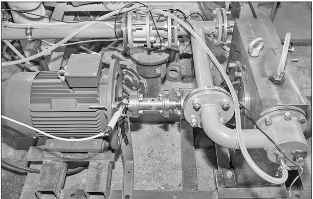
Турбодетандер сумських науковців дає змогу перетворювати стиснену енергію пару, яка виникає під час розподілу газу, на електроенергію
