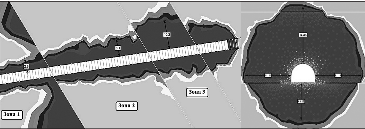
Комп'ютерне моделювання переходу тектонічного порушення. Поздовжній та поперечний перетини квершлягу та зони зруйнованих порід навколо нього під час проходження Богданівського скиду
