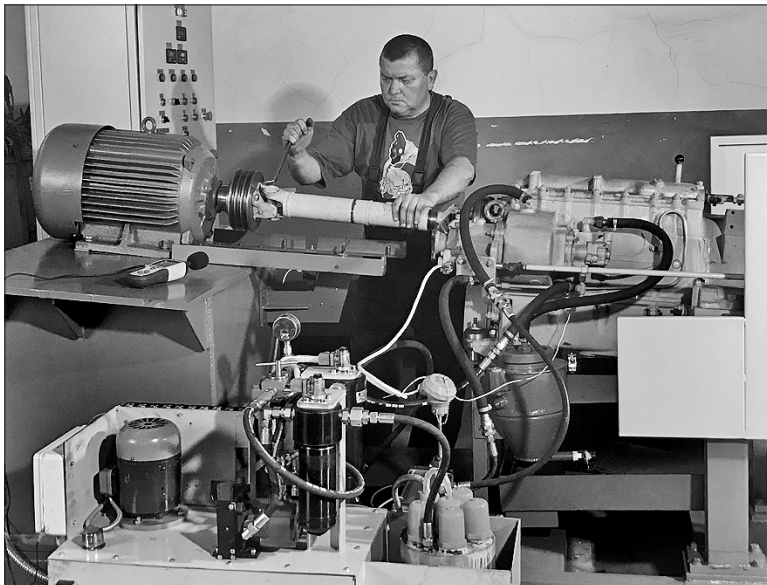
Стендові випробування комплектуючих для бронетанкової техніки
