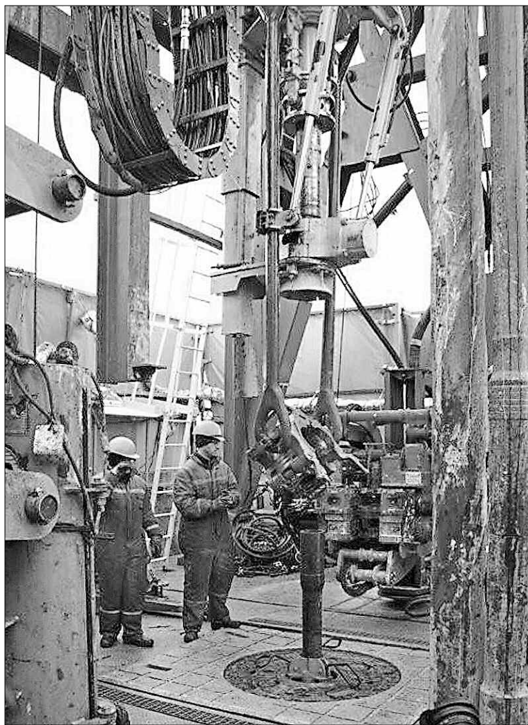
Буріння газової свердловини на Мехедівсько-Голотовщинському родовищі (Лохвицький р-н Полтавської обл.)
