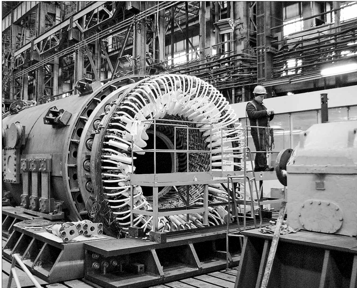
Виготовлення турбогенератора потужністю 550 мегават для Екібастузської ГРЕС
