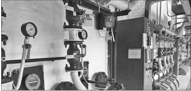
Сучасну котельню обладнано приладами обліку та контролю
